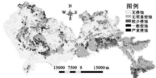
图 2 深圳市 2004 年土壤侵蚀分布图
