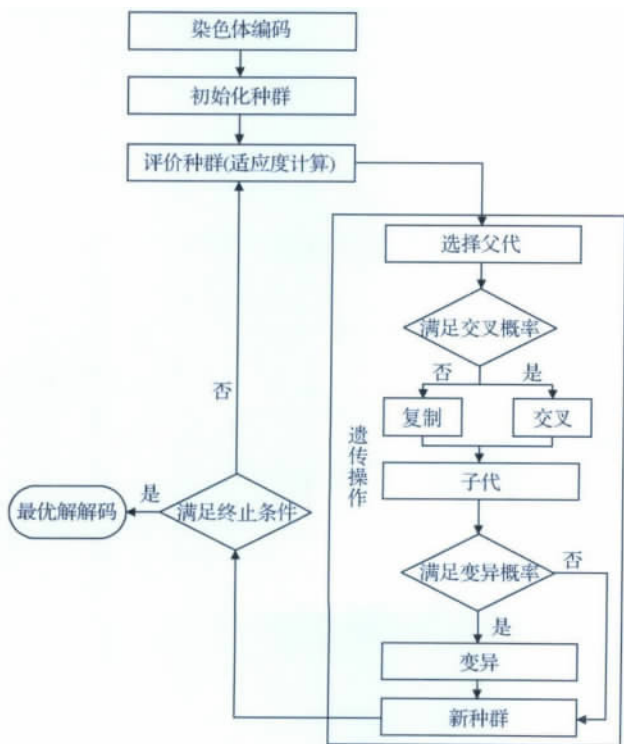
图 4 遗传算法流程图
