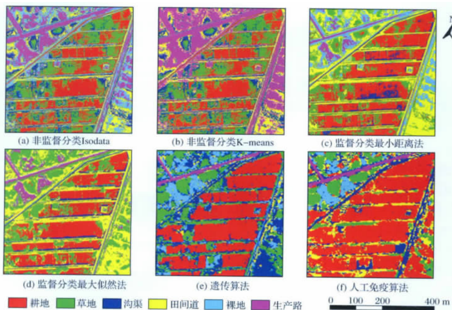
图 7 分类结果图
