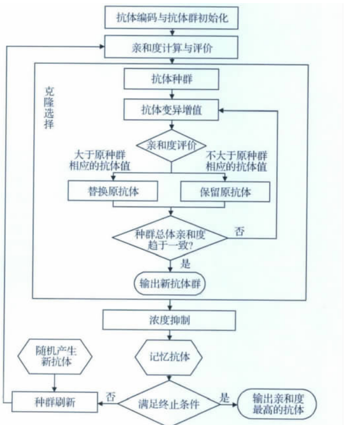
图 5 人工免疫算法流程图
