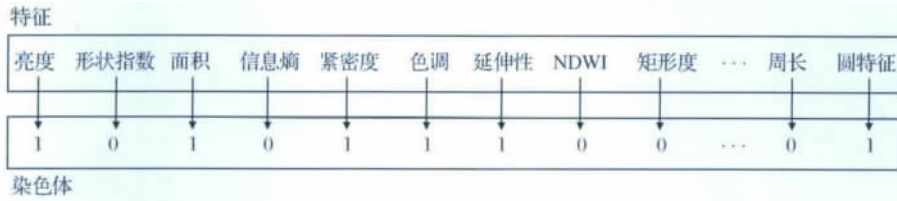
图 3 染色体编码
